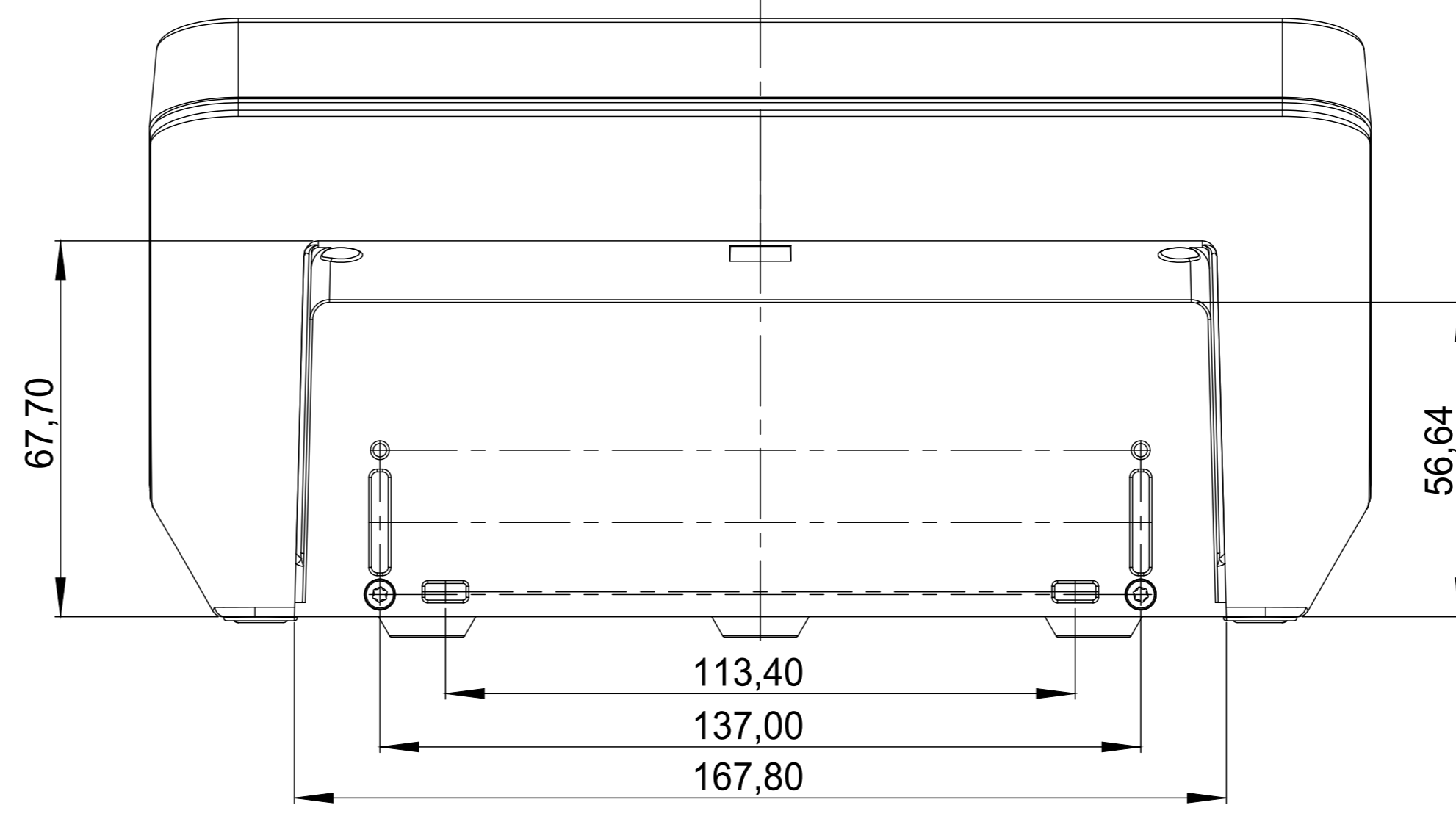
Platine Oberteil P C B Top Part
