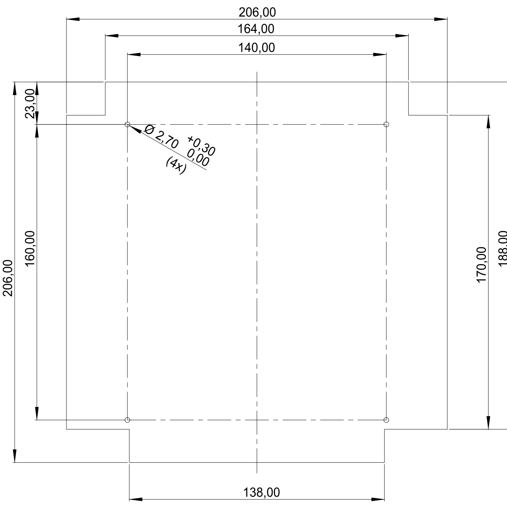
Platine Oberteil P C B Top Part
