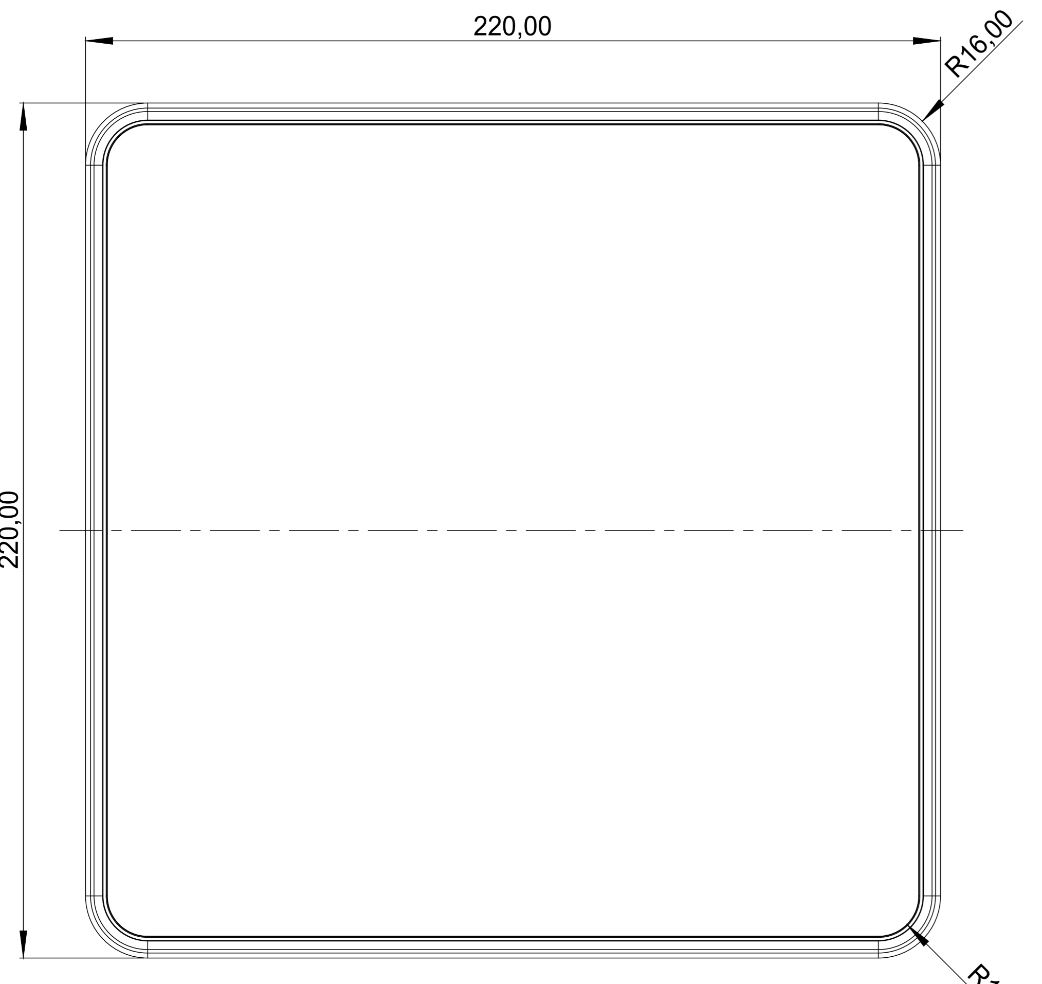
Oberteil Top Part
