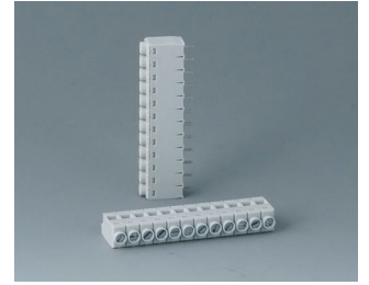
B6603111 Клеммная колодка, шаг 5,0 мм ПА 68 (UL 94 V-0)
