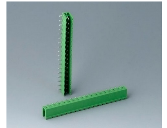
B6604222 Вилочная часть соединителя, шаг 5,08 мм ПА 68 (UL 94 V-0)
