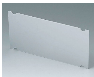
A9195301 Лицевая панель 150 A Алюминий матово-анодированный 141,8x71,6x1,5mm
