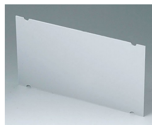
A9195401 Лицевая панель 210 A Алюминий матово-анодированный 201x116x1,5mm
