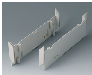
B2030107 Боковые панели для ручки 220, с отверстиями для ручки АБС (UL 94 HB) белый RAL 9002
