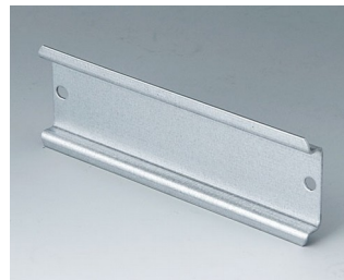
C7112077 DIN-рейка TH 35 Сталь 108x35x7,5mm
