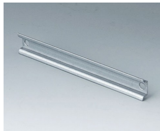
C7111087 DIN-рейка TH 15 Сталь 104x15x5,5mm
