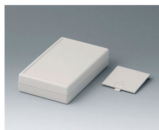
A9408757 SHELL-TYPE CASE G 155, исп. V АБС (UL 94 HB) белый RAL 9002 95x158x33,5mm
